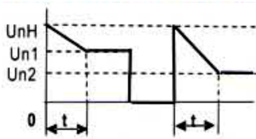
Толчковый пуск
