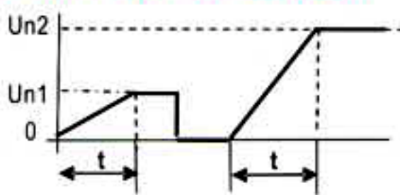
Плавный пуск
